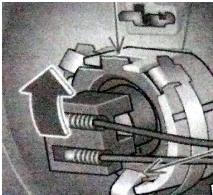
Bild 1: Glühlampenverrastung
